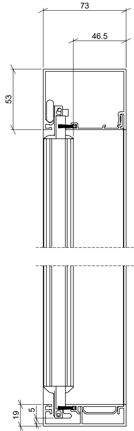
SECTION A-A
